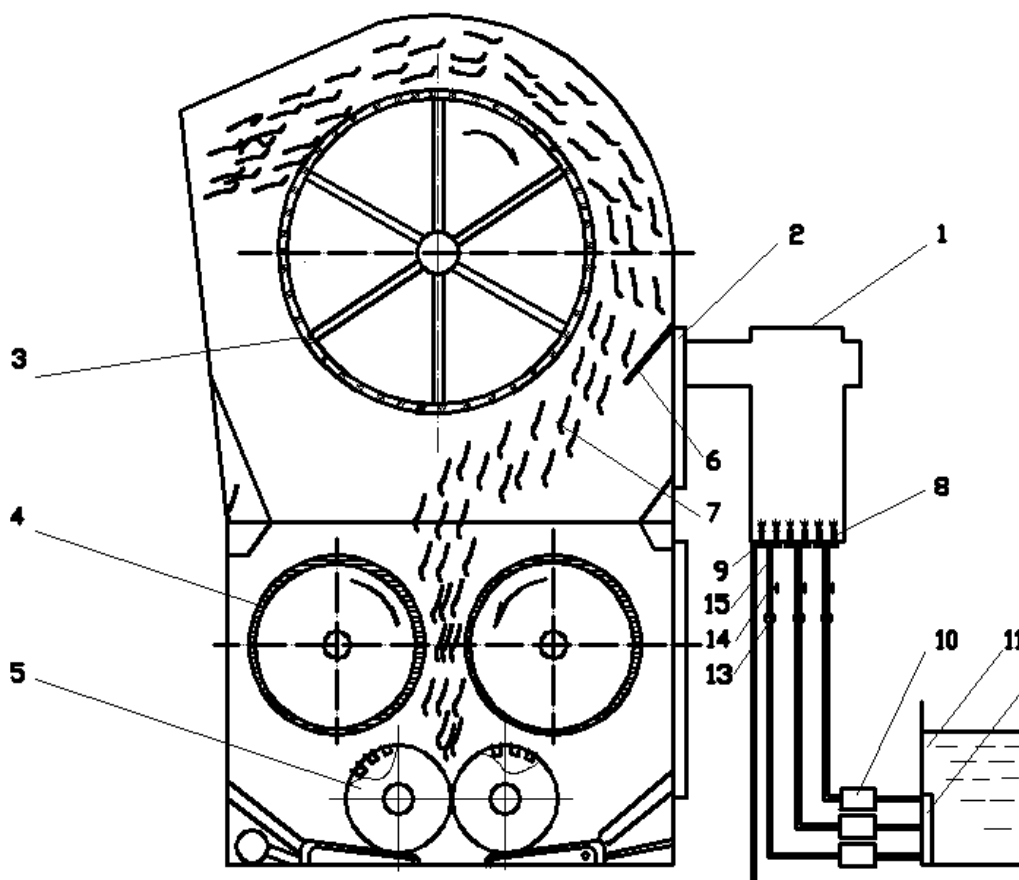
1-rasm. Tolali namlagichli kondensatorning sxematik ko'rinishi
