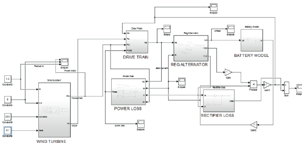
Рисунок 8. Simulink-модель структуры системы.
