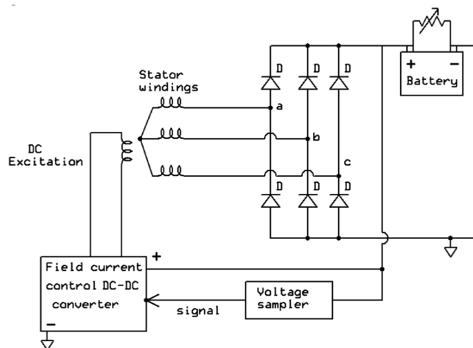
Рисунок 7. Схема системы.
