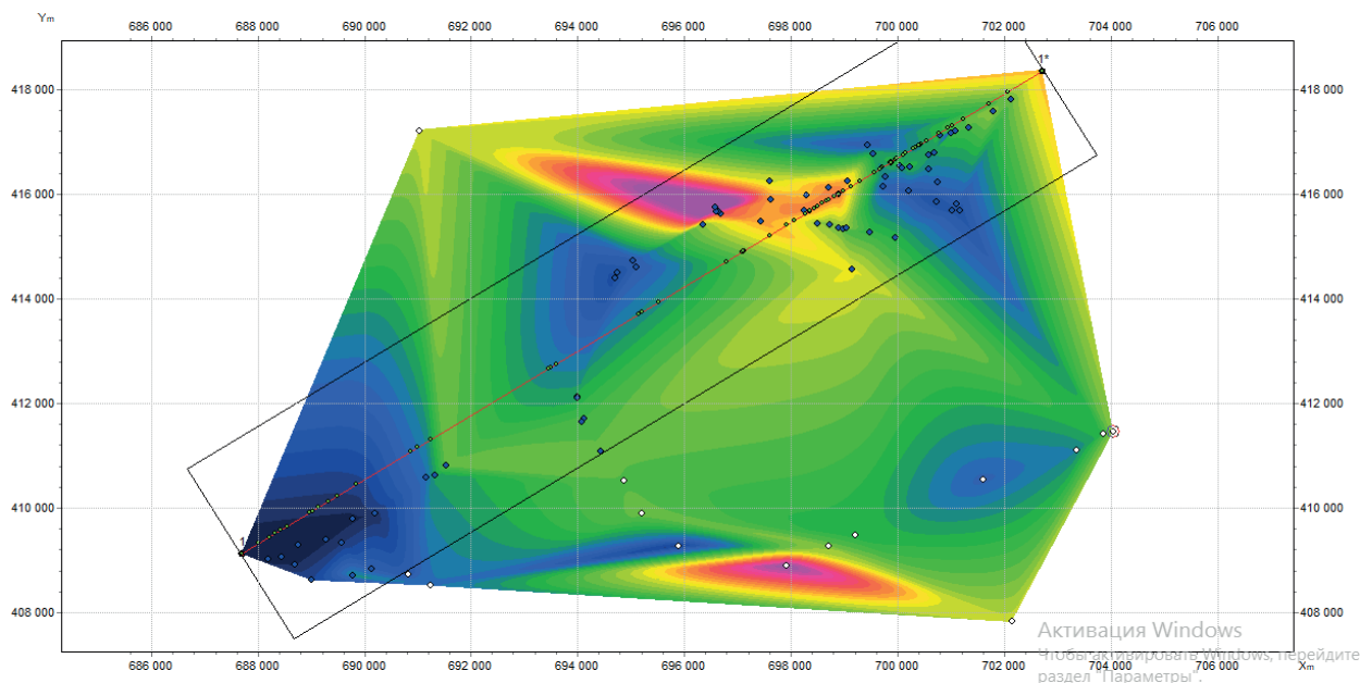
Рисунок 2. Карта магнитного поля Янгибазарское научно-исследовательское геофизическое обсерватория и его ближайшие территории
