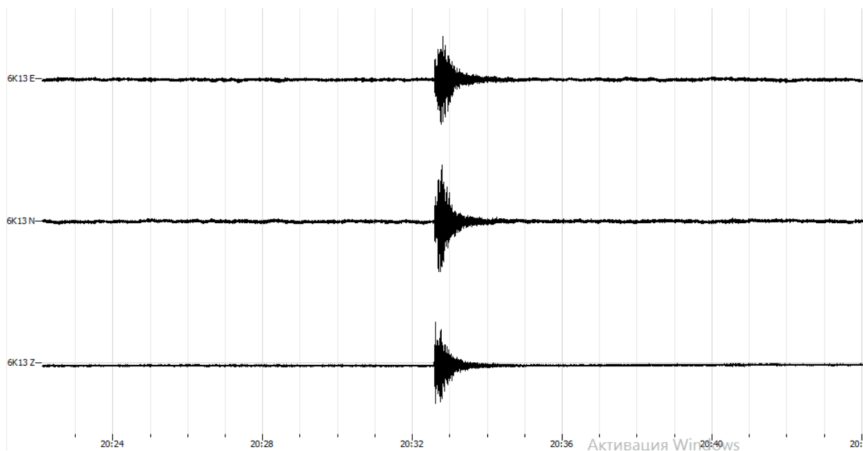
Рисунок 4. Запись землетрясения Янгибазарская станция 19.10.2024 года 01:32 времени Эпицентр: Ташкентская область, Уртачирчикский район.
